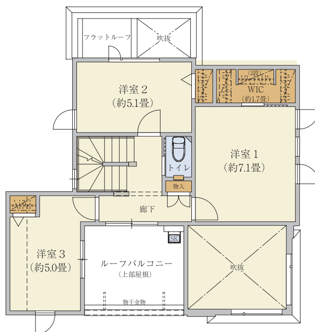
【2階平面図】
