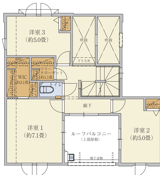
【2階平面図】
