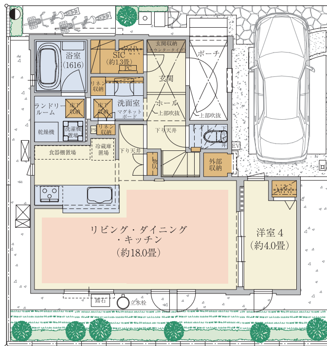
【1階平面図】
