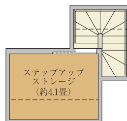
【2階平面図】
