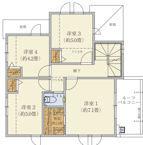
【2階平面図】
