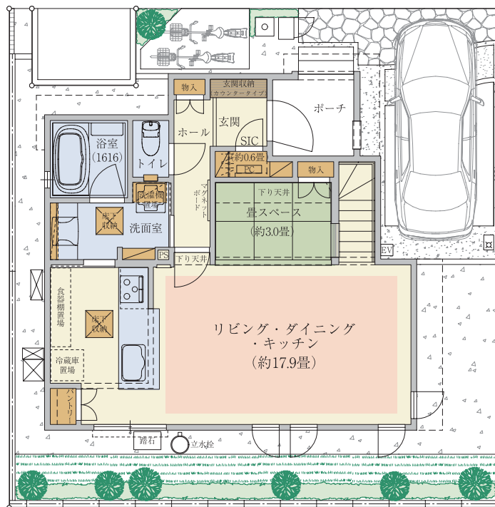
【1階平面図】
