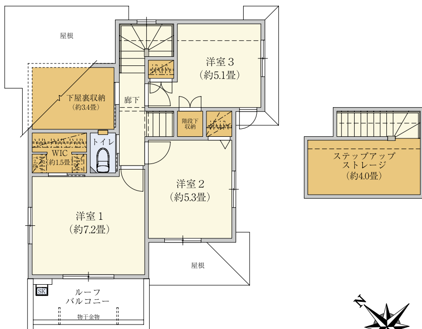
【2階平面図】
