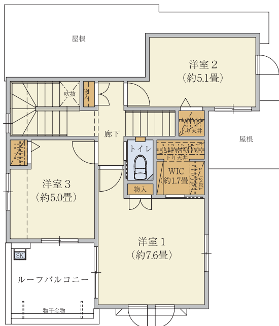
【2階平面図】
