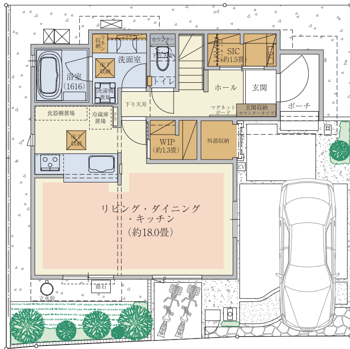
【1階平面図】
