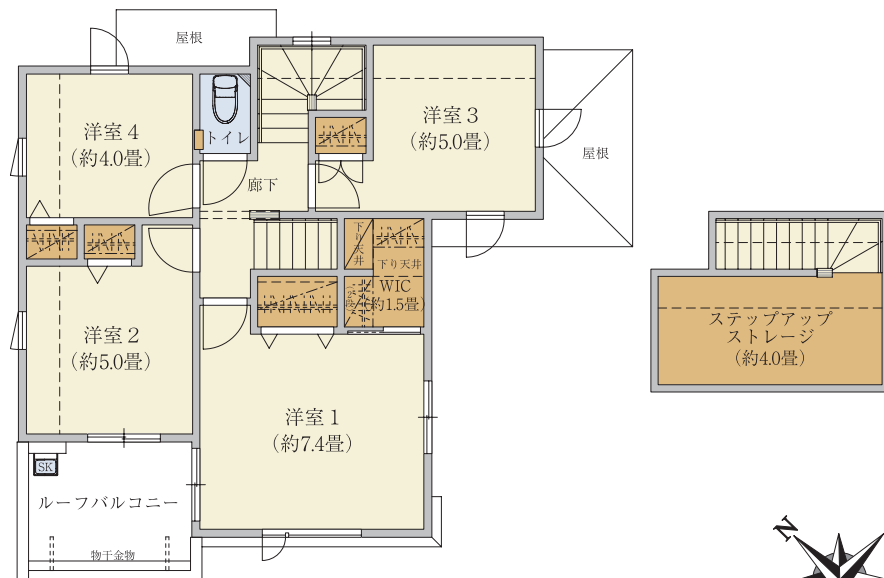
【2階平面図】
