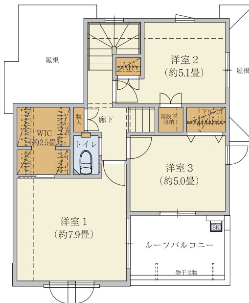
【2階平面図】
