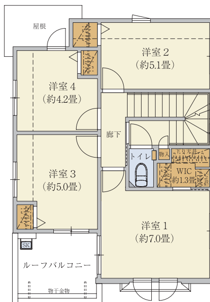
【2階平面図】
