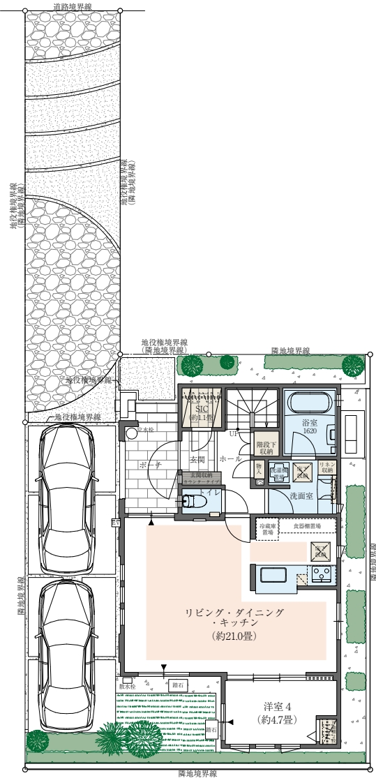
【1階平面図】
