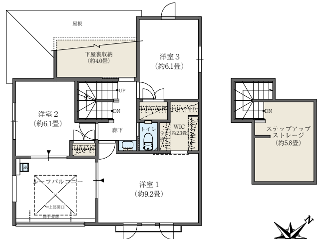
【2階平面図】
