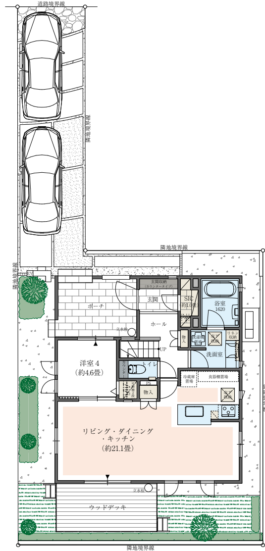
【1階平面図】
